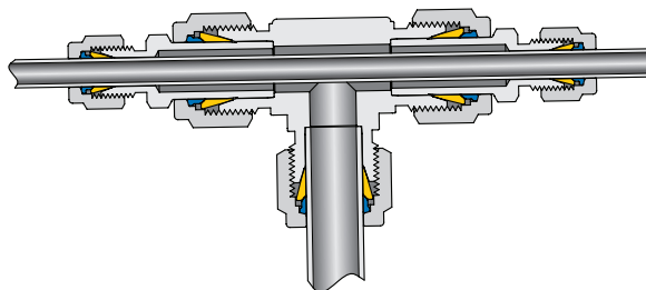
LET-LOK®チューブ継手で組み立てた熱交換器用ティ
